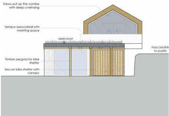
Elevation C-C
