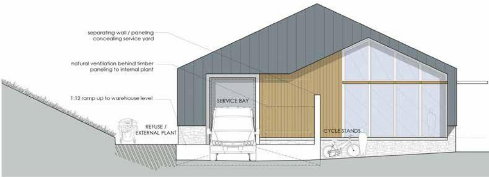
Elevation C-C
